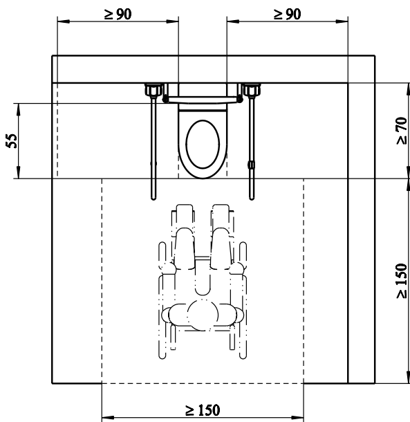
Normgerecht DIN 18040-1
